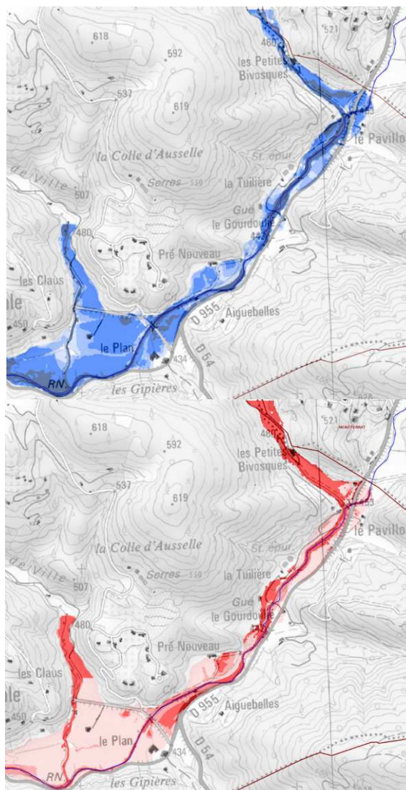
Figure 24 : Hauteur d'eau et vitesses d'écoulement – Le plan
